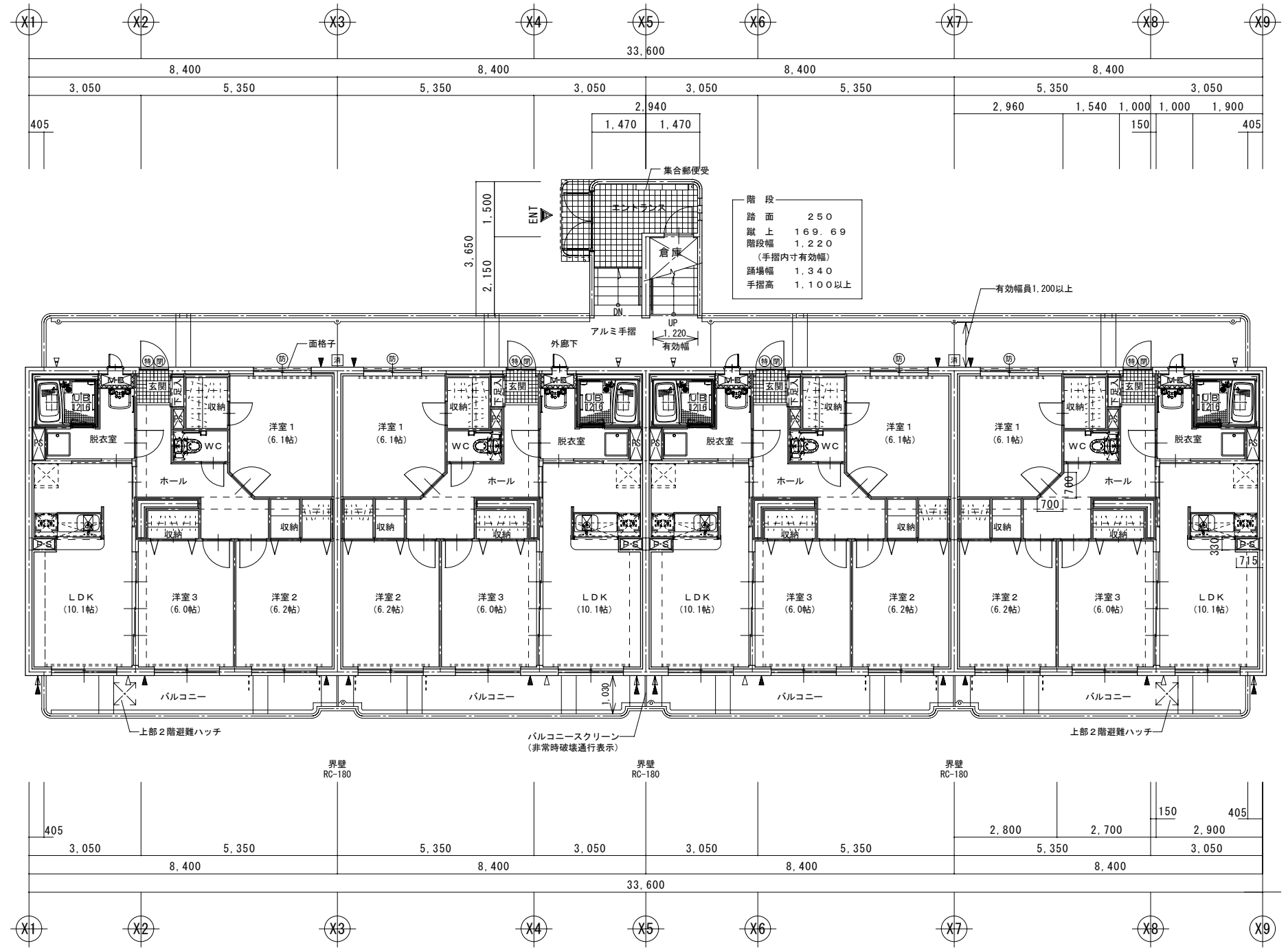
1階平面図 SCALE = 1:100
