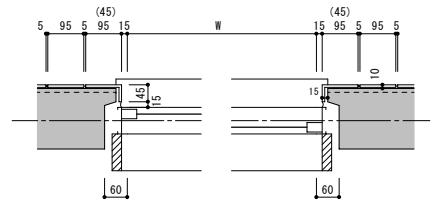
AWサッシュ納まり詳細図 (タイル貼) S=1/10
