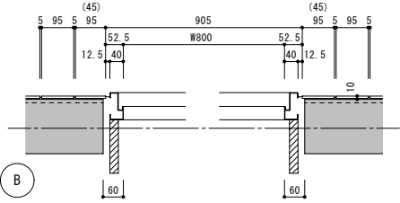
SD-1サッシュ納まり詳細図 (タイル貼) S=1/10
