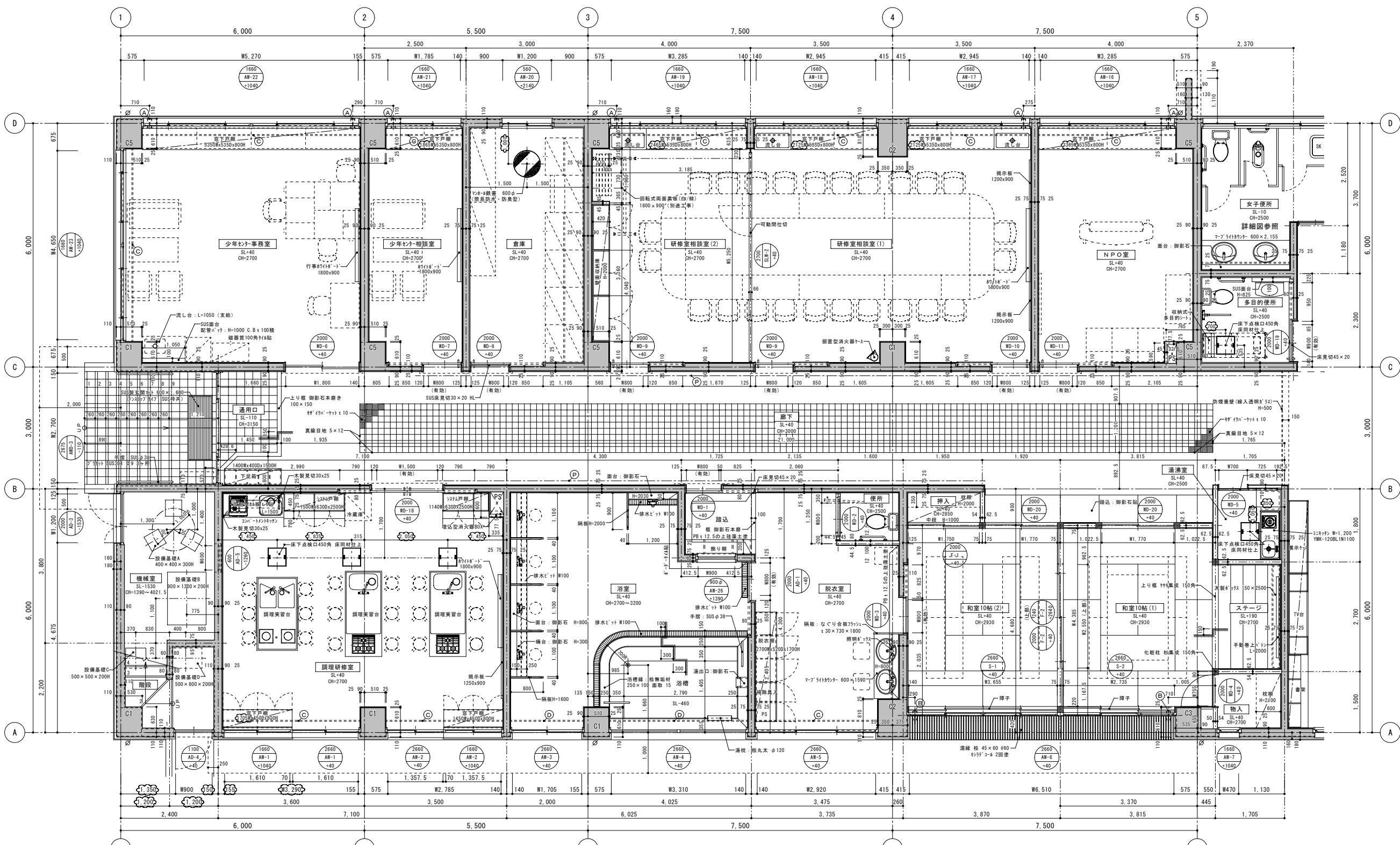
1階平面詳細図(1) S=1/50
